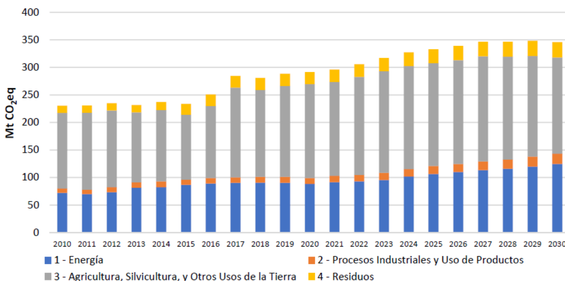
Figura 8. Escenario de referencia para las emisiones de gases de efecto invernadero en Colombia
