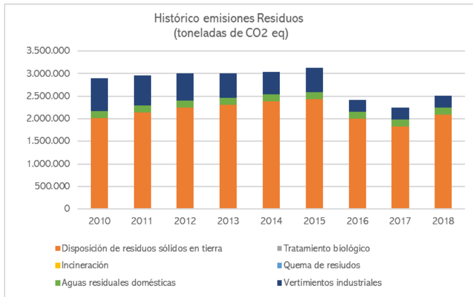
Figura 121. Emisiones históricas por disposición final de los residuos sólidos en Bogotá (toneladas CO 2 eq)
