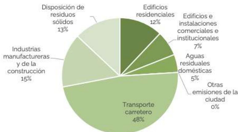
Figura 18. Distribución porcentual de las emisiones GEI por subsector
