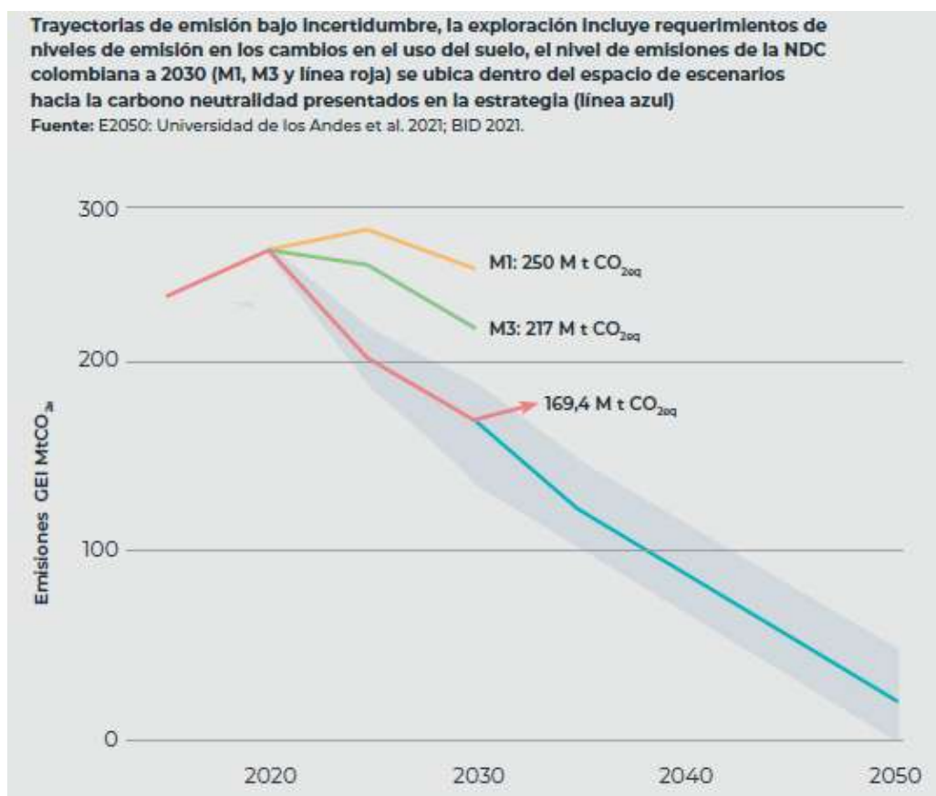
Figura 9. Trayectorias de emisión de Colombia bajo incertidumbre
