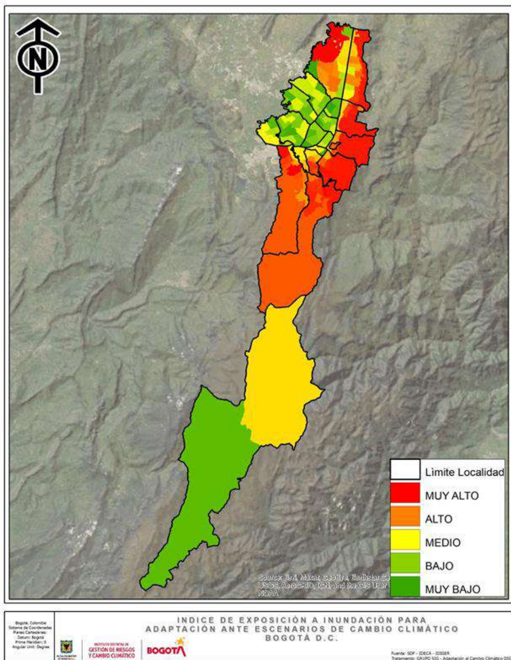
Figura 27. Índice de exposición por inundación para adaptación ante escenarios de cambio climático
