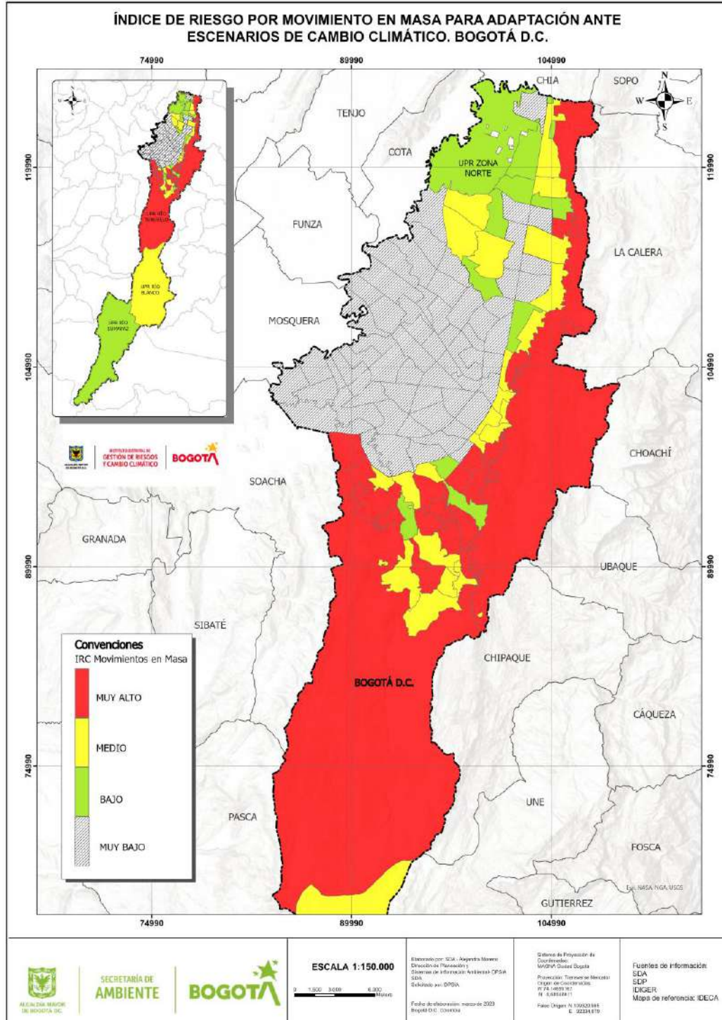
Figura 33. IRC por movimientos en masa
