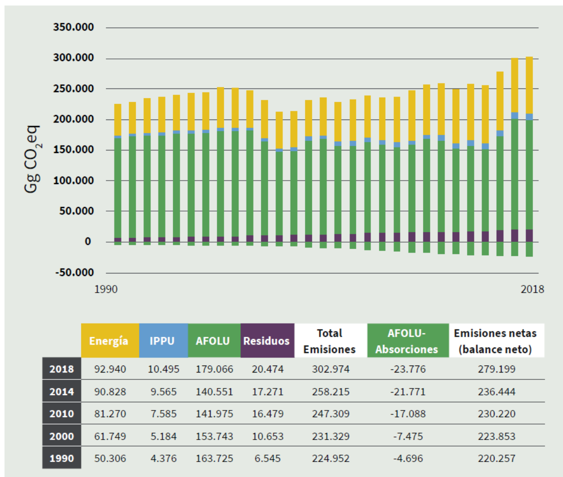
Figura 7. Inventario Nacional de Emisiones y Absorciones de GEI de Colombia serie 1990-2018
