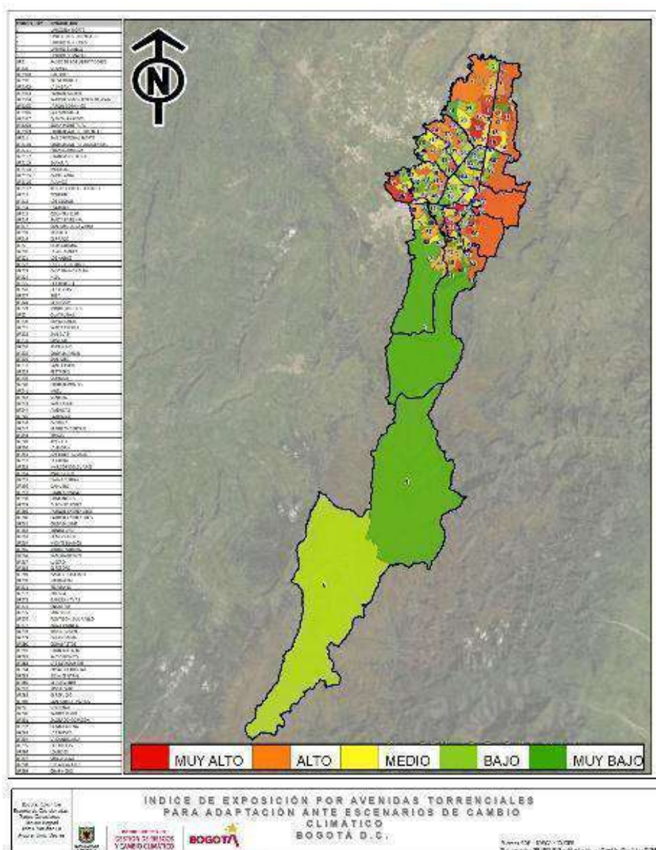
Figura 43. Índice de exposición por avenidas torrenciales para adaptación ante escenarios de cambio climático
