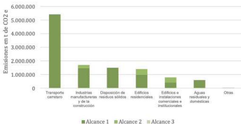
Figura 19. Emisiones por subsector y por alcance
