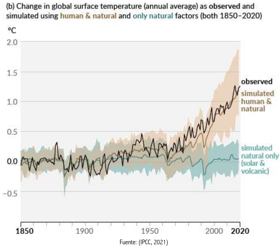
Figura 5. Cambio en el promedio anual de la temperatura superficial: medido, simulado con contribuciones naturales y simulado con contribuciones naturales y humanas combinadas
