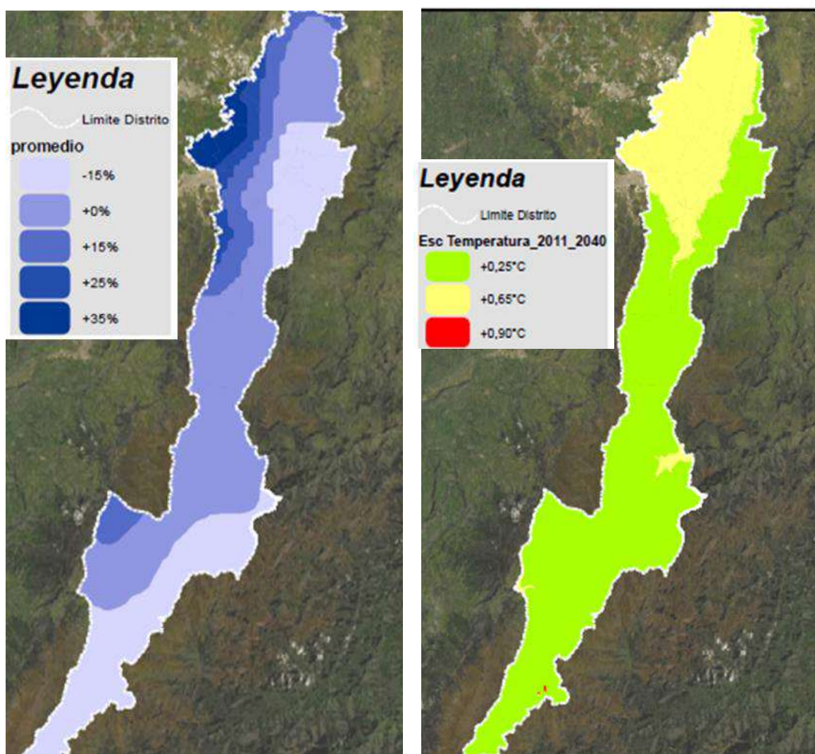
Figura 24. Escenario de aumento de la temperatura media anual en grados centígrados (derecha) y escenario de cambio en las lluvias en porcentaje (izquierda)
