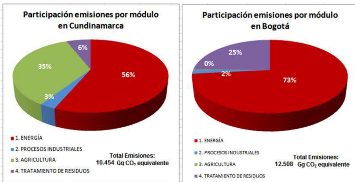
Figura 10. Participación por módulo sobre el total de emisiones en Gg de CO 2 equivalente para Bogotá y Cundinamarca.
