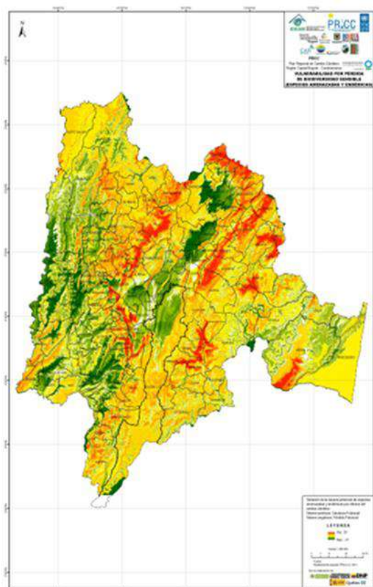
Figura 11. Vulnerabilidad por pérdida de biodiversidad sensible (especies amenazadas y endémicas) por efectos del cambio climático
