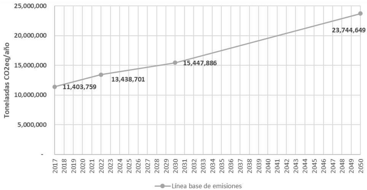
Figura 20. Trayectoria de emisiones en el escenario BAU desde 2017 a 2050
