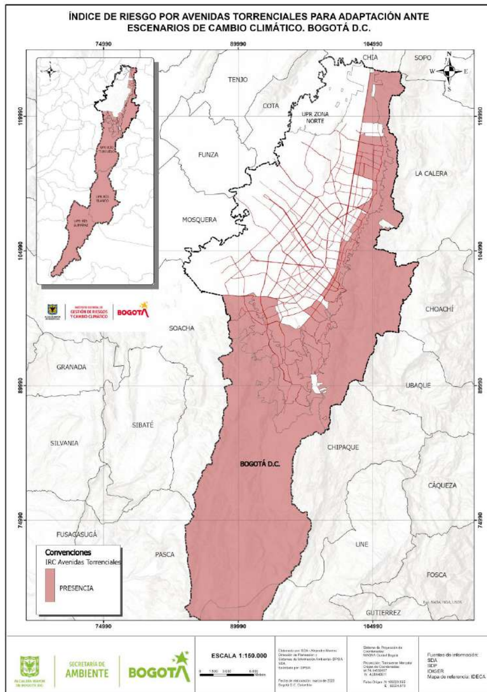
Figura 42. IRC avenidas torrenciales
