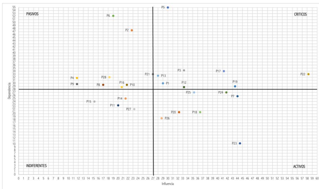
Figura 129. Plano cartesiano - Vester
