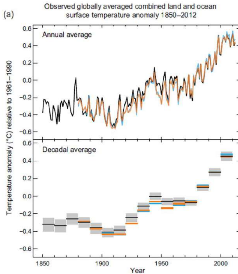
Figura 4. Anomalías en la temperatura media global combinada de las superficies de océano y tierra.
