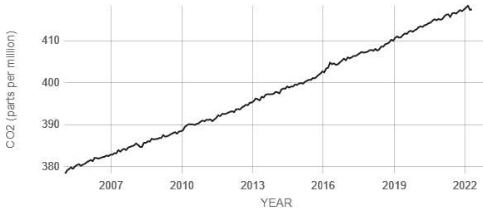
Figura 3. Concentración histórica de CO 2 en la atmósfera. Promedio de las mediciones directas (se ha removido la variación estacional) realizadas en el observatorio Mauna Loa (Hawaii) en los últimos años
