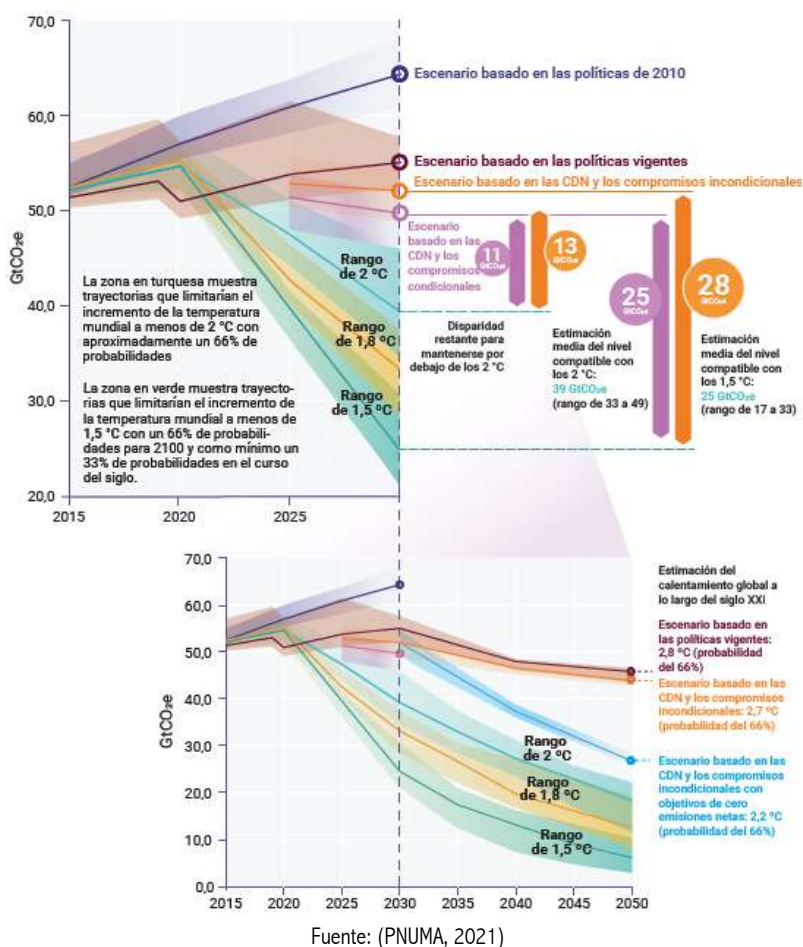
Figura 127. Emisiones mundiales de gases de efecto invernadero para diferentes escenarios y estimación de las desviaciones con respecto al logro de los objetivos climáticos
