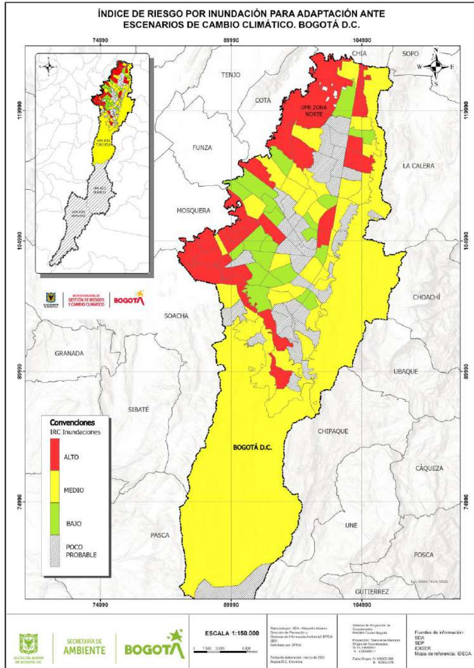
Figura 28. IRC por inundación
