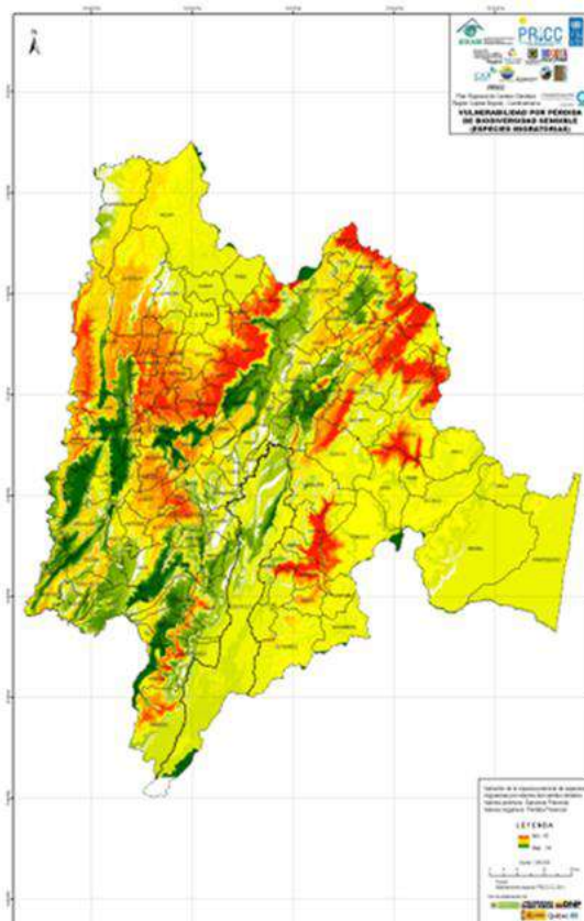
Figura 12. Vulnerabilidad por pérdida de biodiversidad sensible (especies migratorias) por efectos del cambio climático.
