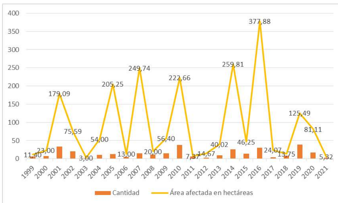
Figura 34. Cantidad de incendios forestales reportados por año en Bogotá D.C., entre 1999 y 2021 y área afectada
