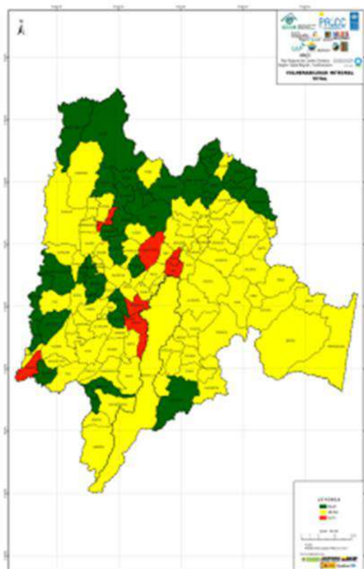
Figura 13. Vulnerabilidad integral total para los municipios del departamento de Cundinamarca
