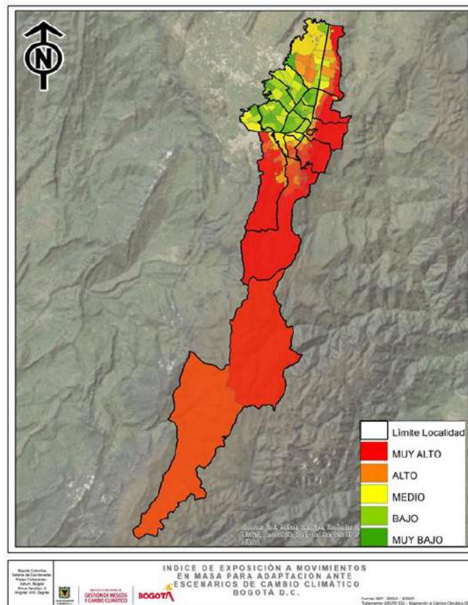
Figura 32. Índice de exposición a movimientos en masa para adaptación ante escenarios de cambio climático
