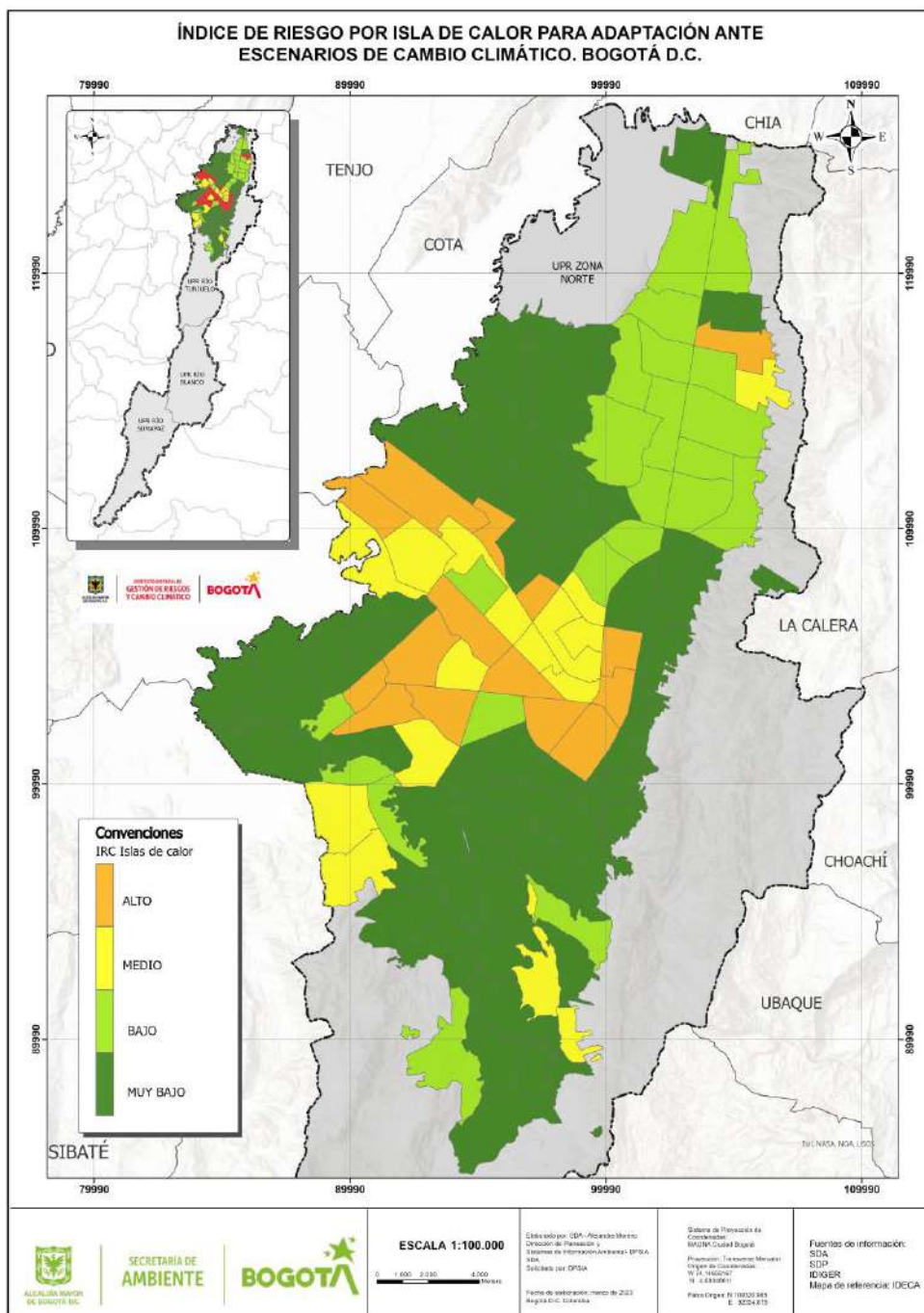
Figura 45. IRC por islas de calor urbanas
