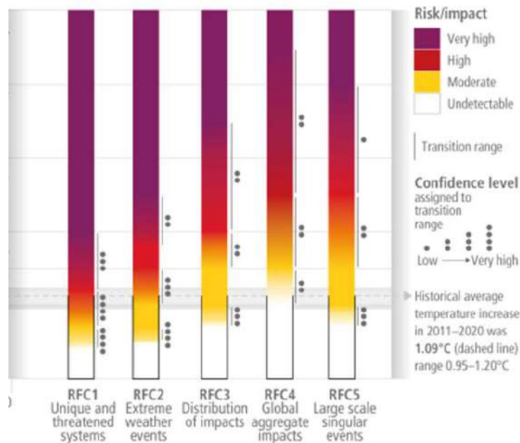
Figura 6. Motivos de preocupación sobre las evaluaciones de impacto y riesgo asumiendo una adaptación baja o nula
