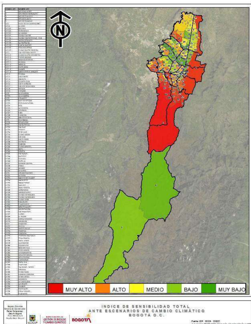
Figura 46. Índice de Sensibilidad Total para la Adaptación ante Escenarios de Cambio Climático Bogotá D.C.
