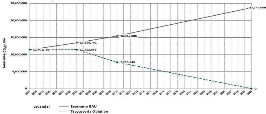
Figura 21. Trayectoria de emisiones en el escenario BAU y escenario de metas de emisión desde 2017 a 2050
