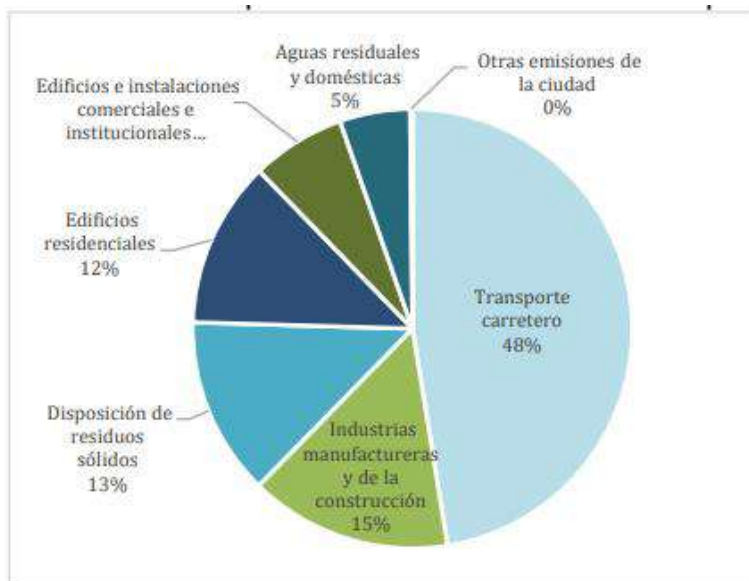
Figura 119. Distribución del aporte de GEI por subsector en Bogotá
