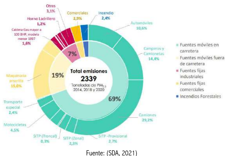
Figura 118. Participación de las fuentes en las emisiones de PM 2.5 por combustión
