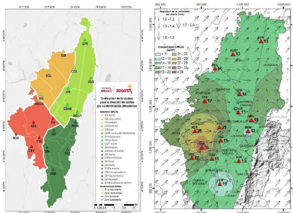
Figura 123. Tendencia interanual de PM_{2.5} en Bogotá 2018-2021. a) Zonificación ambiental y (b) Distribución de PM_{2.5} en la ciudad
