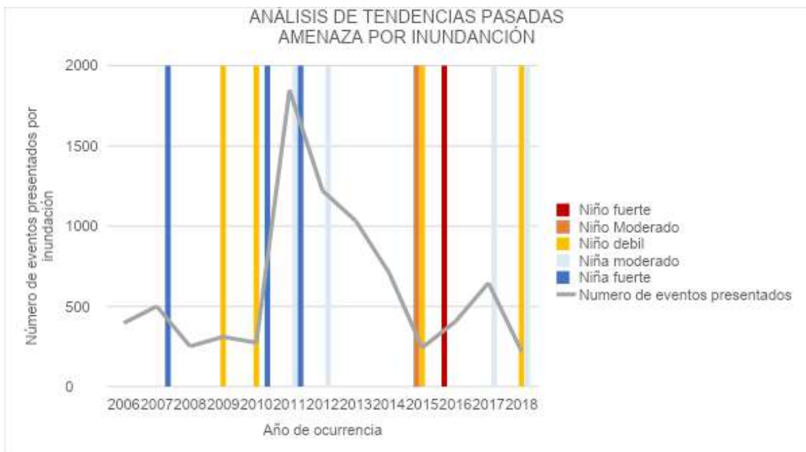
Figura 26. Eventos por inundación (2010-2020)
