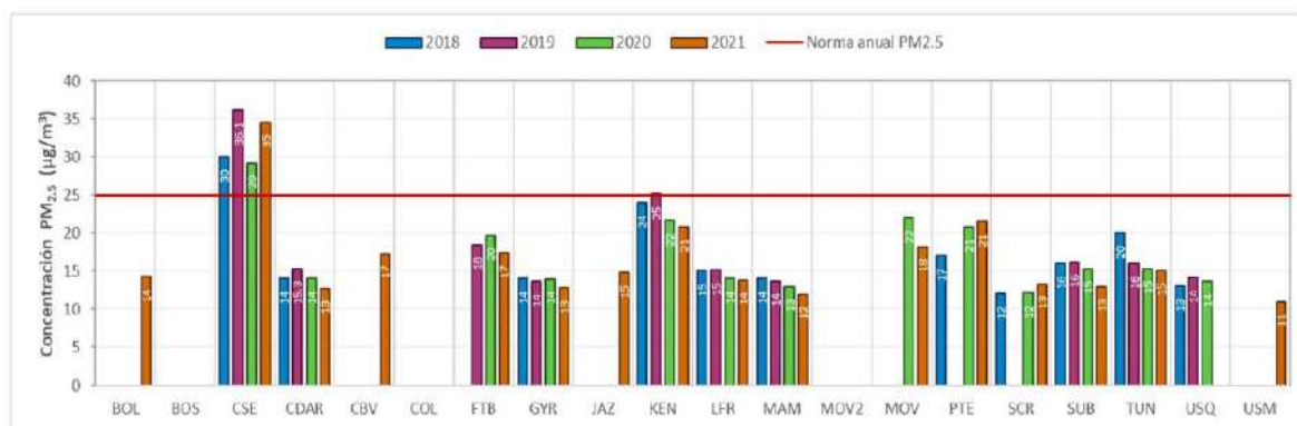
Figura 122. Tendencia interanual de PM_{2.5} en Bogotá 2018-2021.
