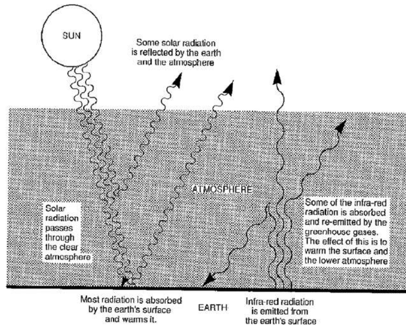
Figura 1. Diagrama simplificado que ilustra el efecto invernadero en el AR1
