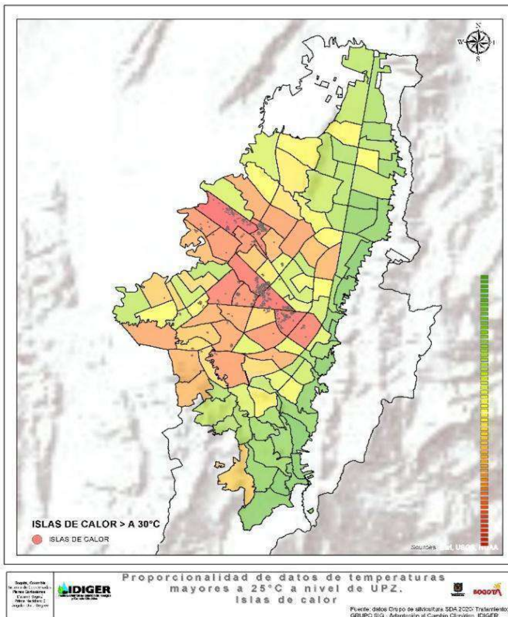
Figura 44. Proporcionalidad de datos de temperatura mayores a 25°C a nivel de UPZ
