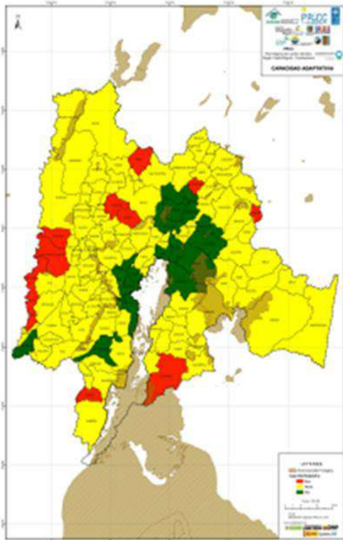
Figura 15. Capacidad de adaptación en el departamento de Cundinamarca
