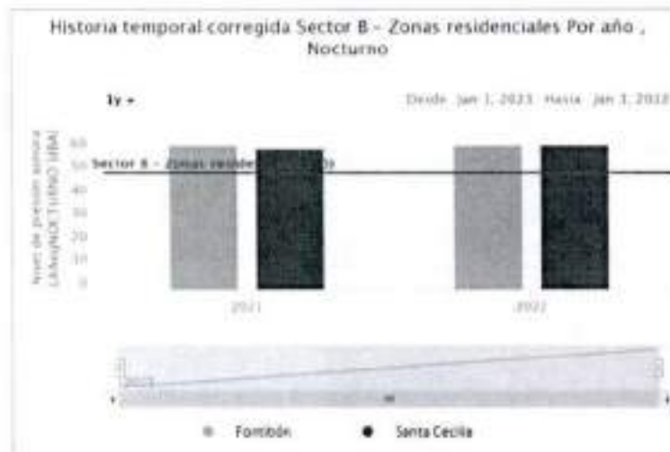
Figura 2. Niveles de presión sonora registrados en Fontibón para el periodo nocturno ( L_p ) Fuente: Área técnica de la Red de Monitoreo de Ruido Ambiental de Bogotá
