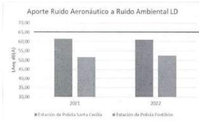
Figura 3. Niveles de presión sonora aeronáuticos en Fontibón para el periodo diurno ( L_D ) Fuente: Área técnica de la Red de Monitoreo de Ruido Ambiental de Bogotá
