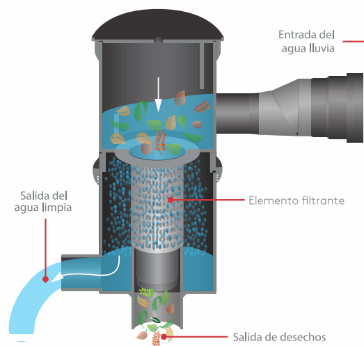
CORTE TRANSVERSAL
